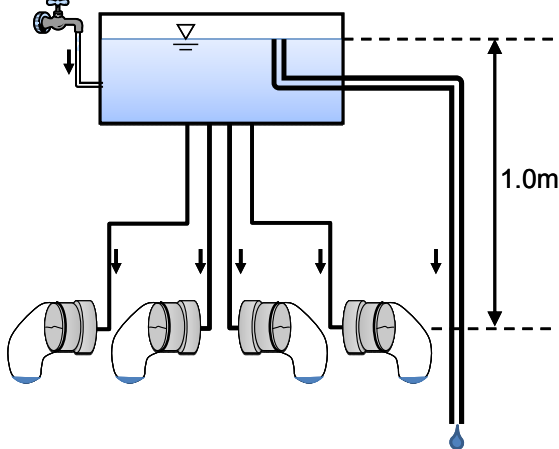
図4 透水試験装置の概要
