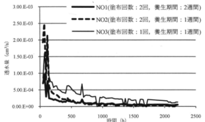
図1 含浸剤塗布後の透水試験結果
