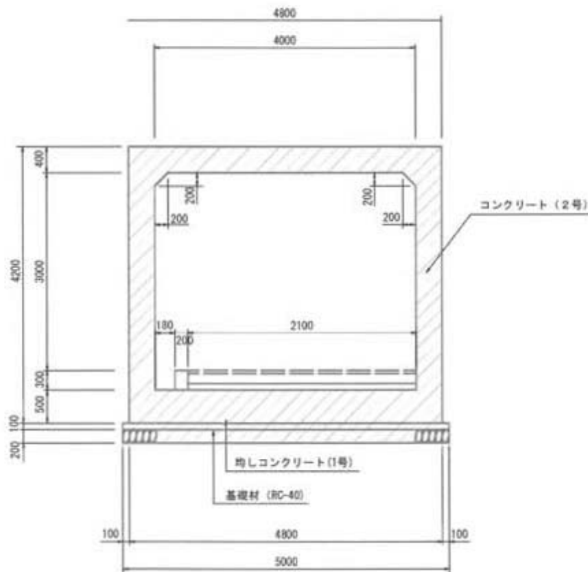
图一-1 地覆部施工(断面图 S=1:50)
