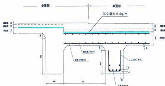
施工概要図
